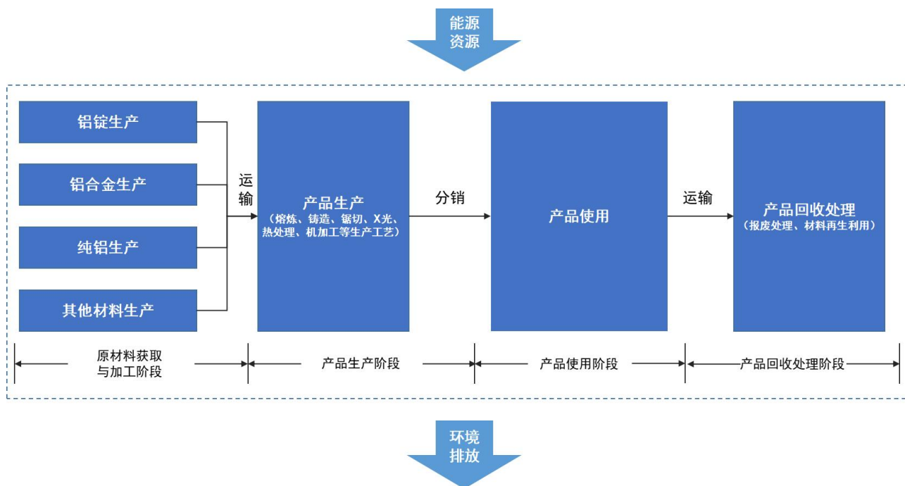
图 4 吉利 KX11 前转向节系统边界图
