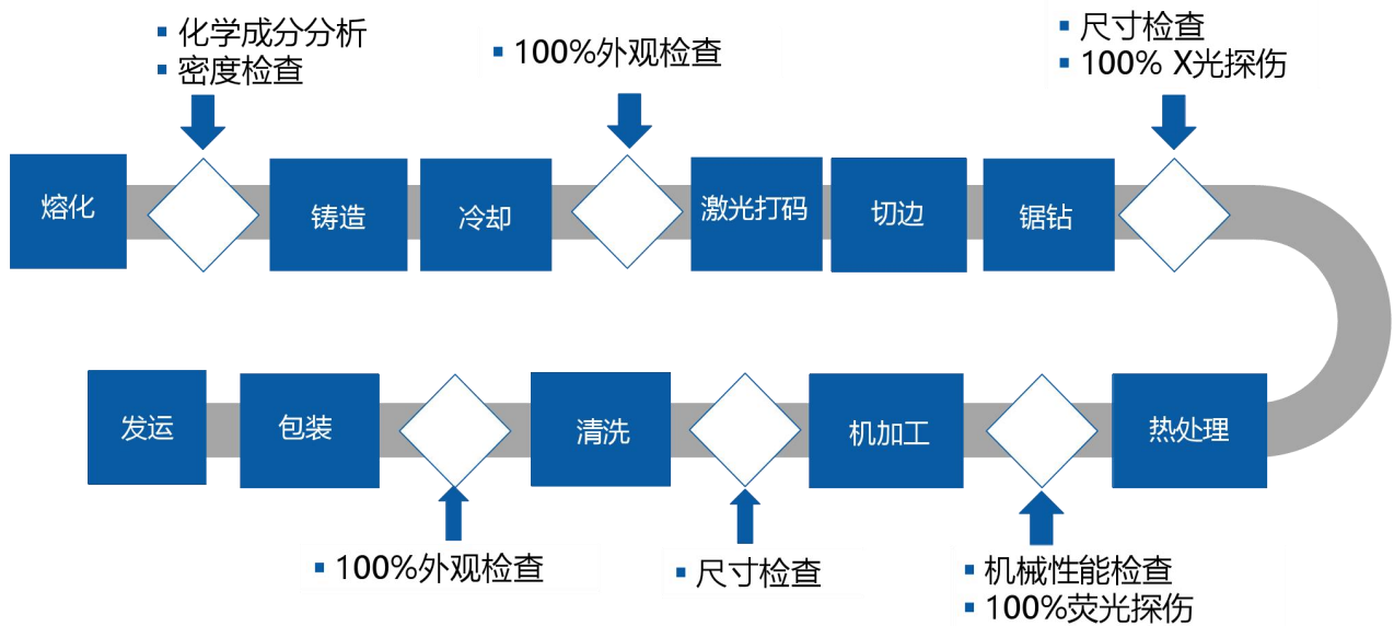
图 6 吉利 KX11 前转向节生产工艺流程图
