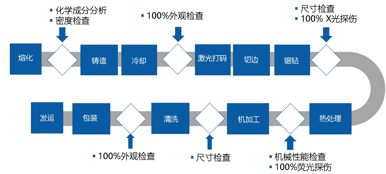
图 B.1 产品生产工艺流程图
